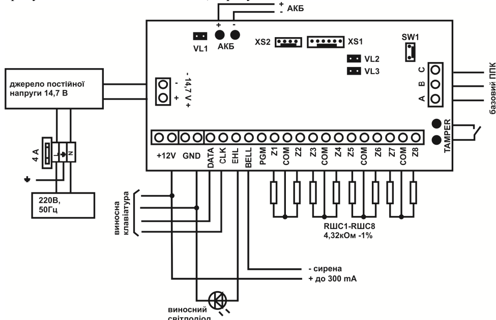
Схема підключення пристрою (Мал. 2)
