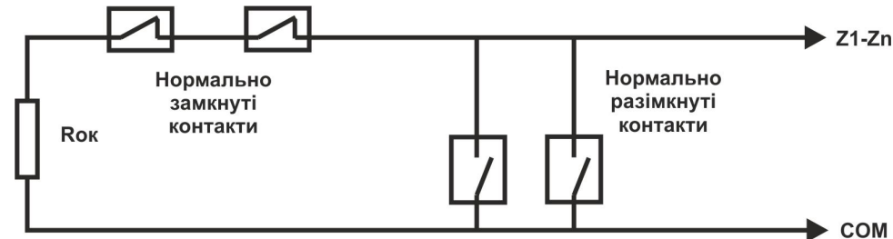
Схема підключення приладу (Мал. 2)
